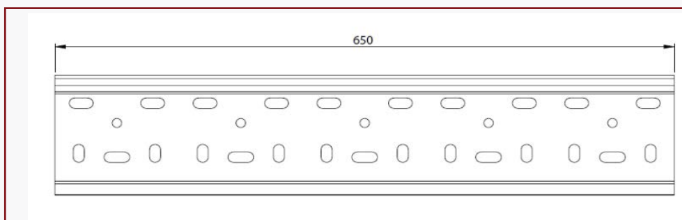
Förlängningskonsol 650mm.
