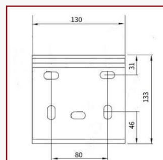
Standardkonsol 130mm
